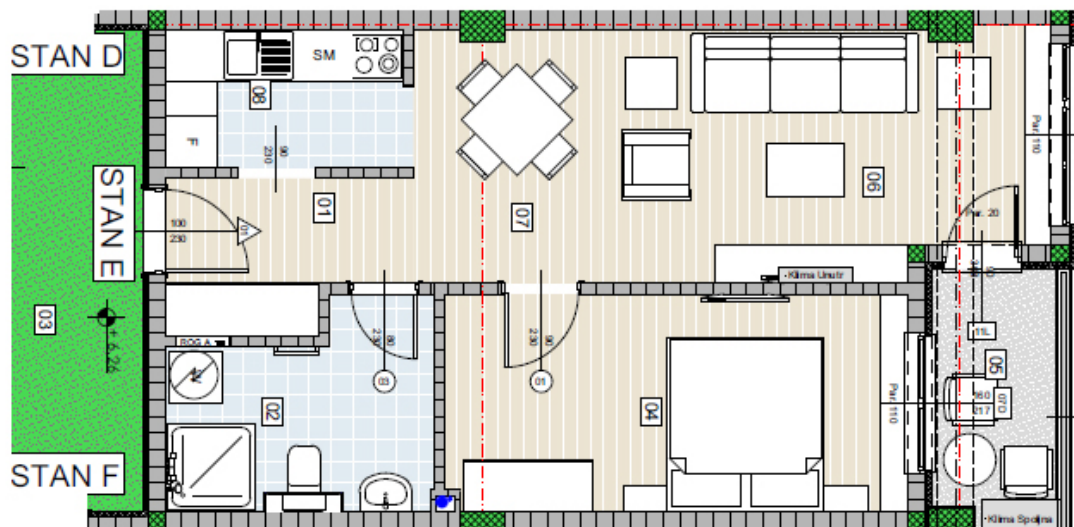
LAMELA A - STAN E - OSNOVA FUNKCIJE R 1:50
