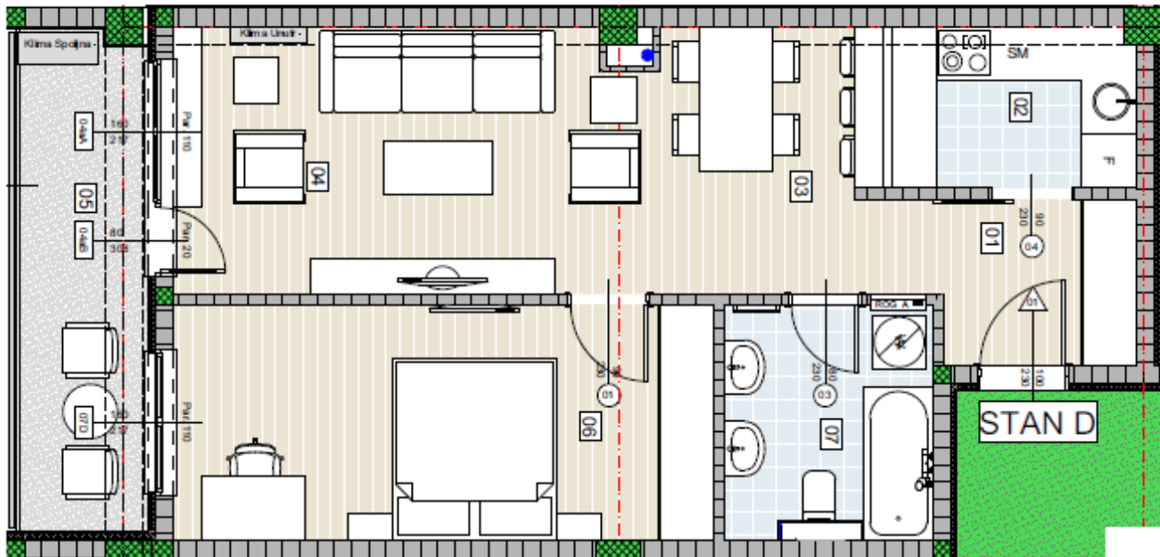
LAMELA D - STAN D - OSNOVA FUNKCIJE R 1:50
