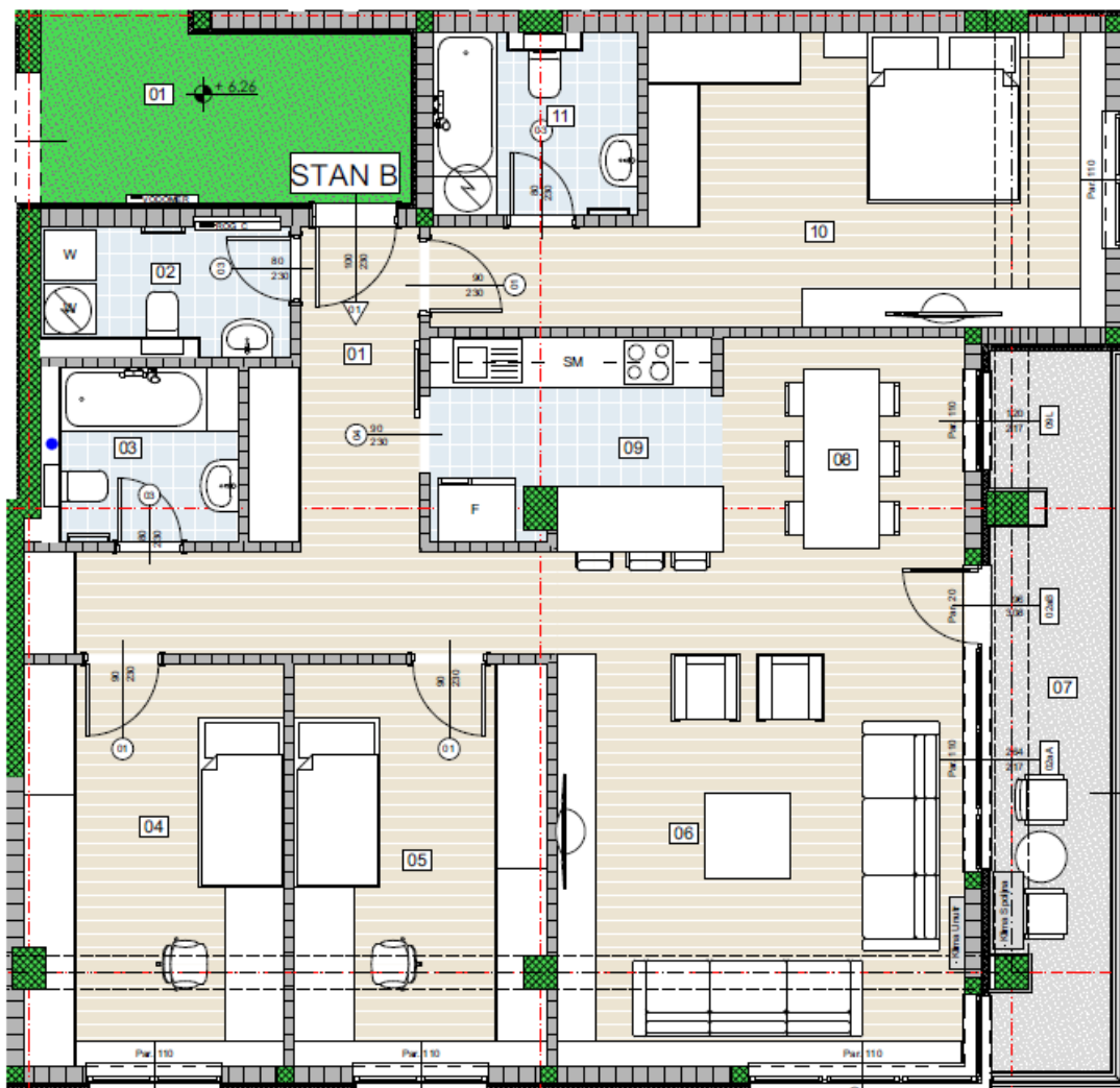
LAMELA C - STAN B - OSNOVA FUNKCIJE R 1:50
